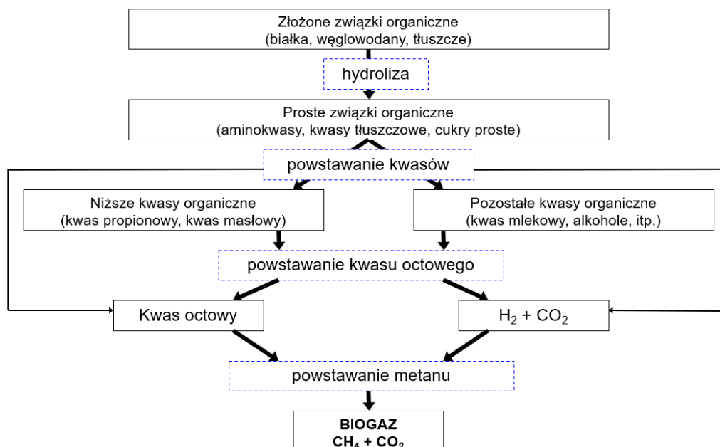
Schemat przebiegu procesów fermentacji metanowej
